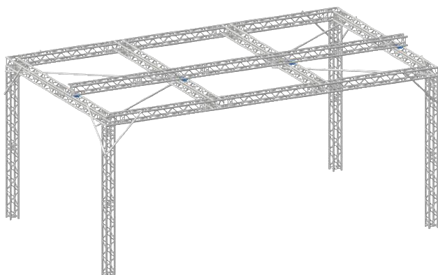
1 Truss System Hoop Scale: 1:50
